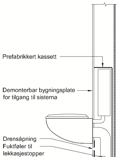
Fig. 3 Prinsippskisse – Installering i tørre rom
