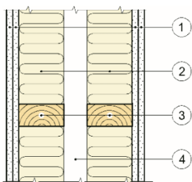
Fig. 4 Prinsipiell oppbygning av lyd- og brannskillevegger
