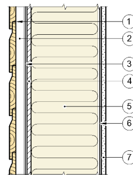
Vertikalsnitt
