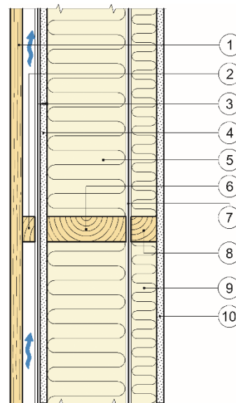
Horisontalsnitt
