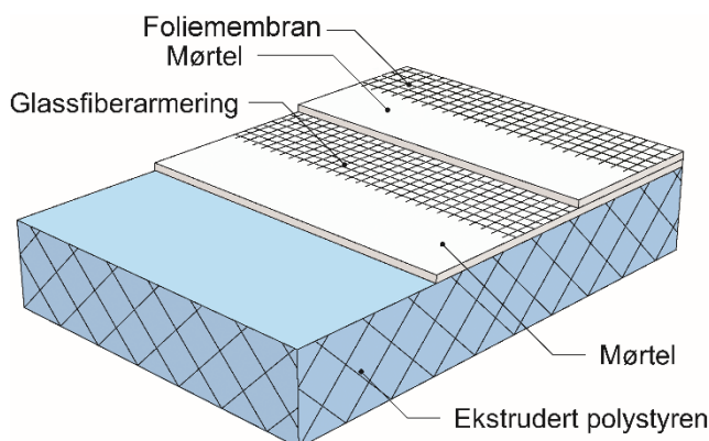
Figur 1. Oppbygningen av wedi Vapor 85 N. Våtromsplatene har armert mørtel på begge sider, og en foliemembran på den ene siden
