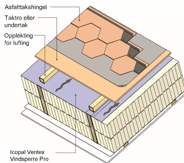
Fig. 2 Eksempel på Icopal Ventex Vindsperre Pro brukt i luftet skrått tak
