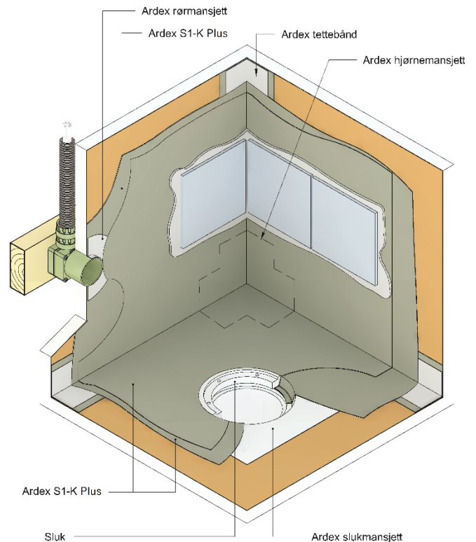
Fig. 1 Oppbygning av Ardex S1-K Plus membransystem
