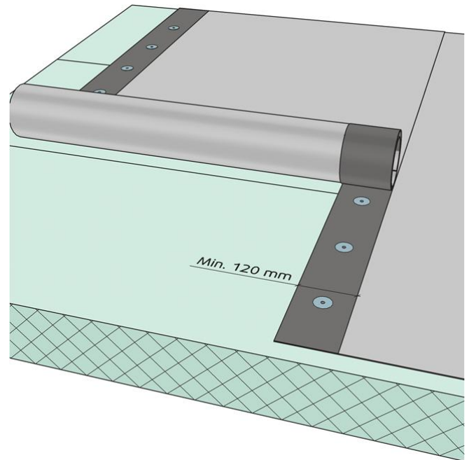
Fig. 1 Norbit Arctic Solo - ettlags asfalt takbelegg legges med minimum 120 mm sveiset omlegg.
