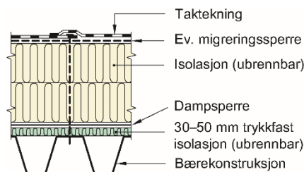
Fig. 2 Siga Dampsperre monterert i kompakt takkonstruksjon
