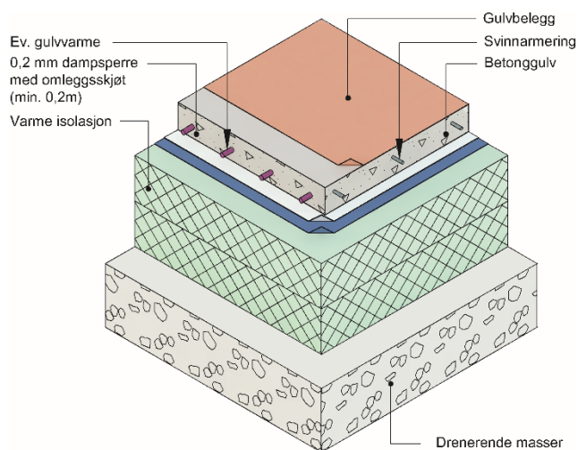
Fig. 3 Siga Dampsperre monterert i betonggolv på grunnen
