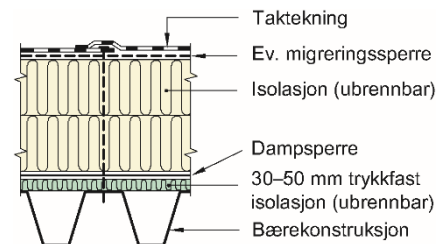
Fig. 2 DAMP ECO monteret i kompakt takkonstruksjon
