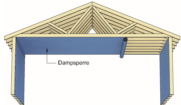
Fig. 1 DAMP ECO monteret i yttervegger og mot kaldt loftsrom
