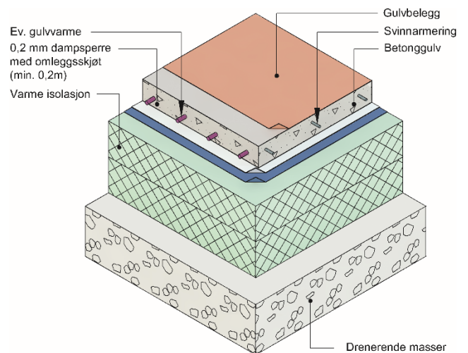
Fig. 3 DAMP ECO monteret i betonggolv på grunnen
