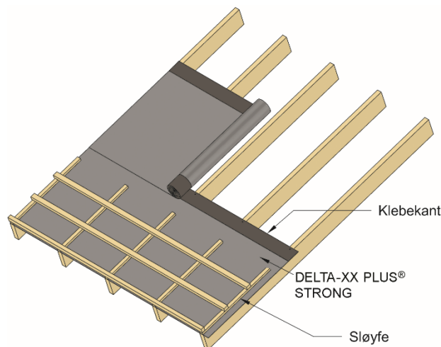
Fig. 1 DELTA-XX PLUS® STRONG kombinert undertak og vindsperre montert tvers av sperrene
