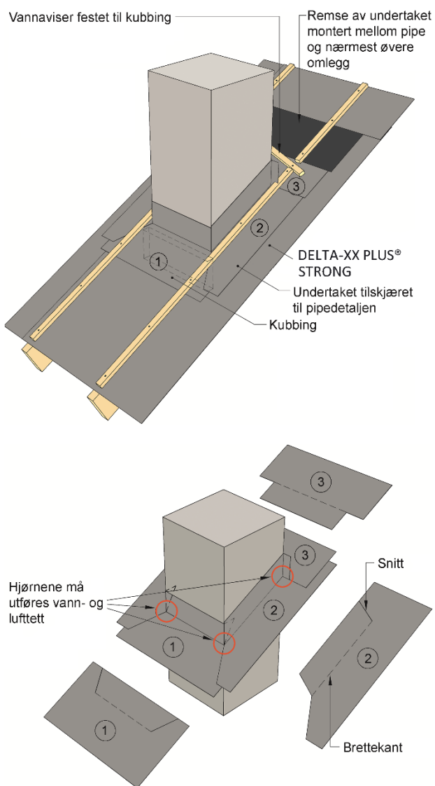
Fig. 5 Eksempel på pipegjennomføring i undertaket. På byggeplass tilskjæres mansjett og monteres ved bruk av klemlakt, DELTA® MULTI-BAND og DELTA® THAN
