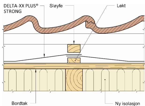
Fig. 6 Eksempel på legging av DELTA-XX PLUS® STRONG på taktro som ikke er plan
