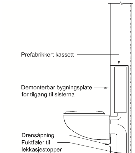
Fig. 3 Prinsippskisse – Installering i tørt rom
