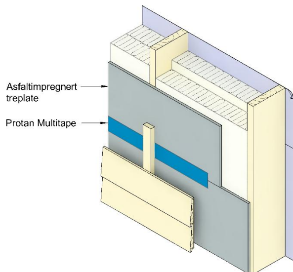
Fig. 2 Eksempel på bruk av Protan Multitape på asfaltimpregnert trefiberplate.
