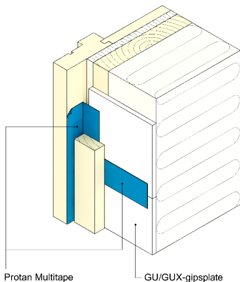
Fig. 3 Eksempel på bruk av Protan Multitape som forsegling av skjøter i vindspærre av GU/GUX gipsplater. Teipen er også brukt som tetting av fuge mellom vindspærre og vinduskarm
