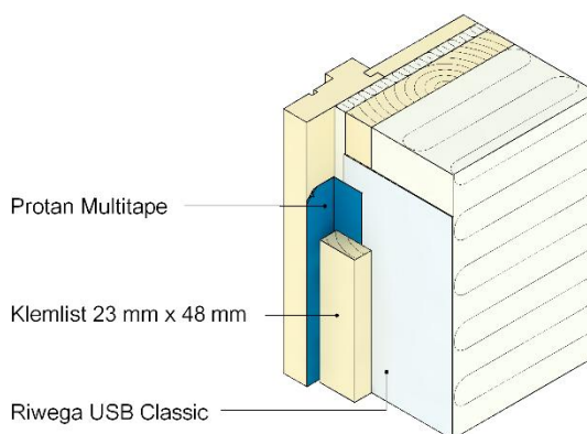
Fig. 1 Eksempel på bruk av Protan Multitape som forsegling av fuge mellom Riwega USB Classic og vinduskarm.
