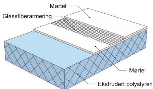
Fig. 1 Oppbygningen av wedi Fundo gulvelementer
