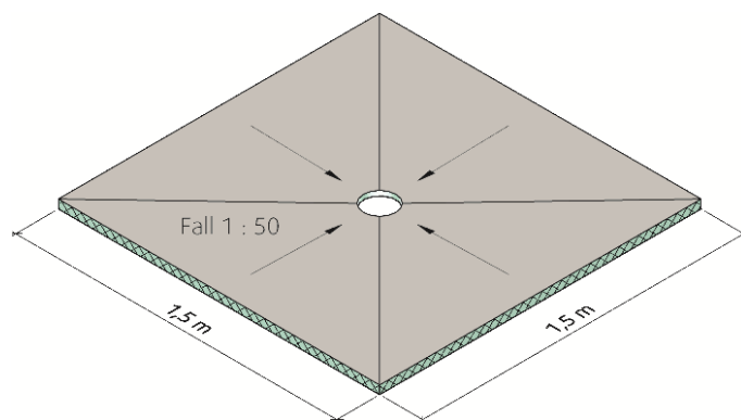
Fig. 2 Eksempel på wedi Fundo gulvelementer med punktavløp sentrert plassert
