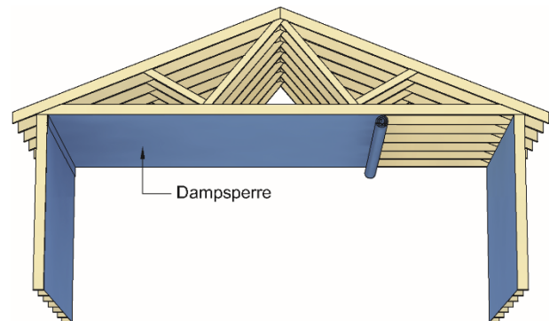
Fig. 1 Kullaplast Dampsperre montert i yttervegger og mot kaldt loftstrom
