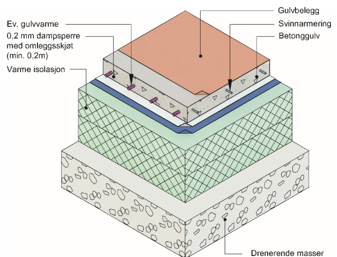
Fig. 3 Kullaplast Dampsperre montert i betonggolv på grunnen
