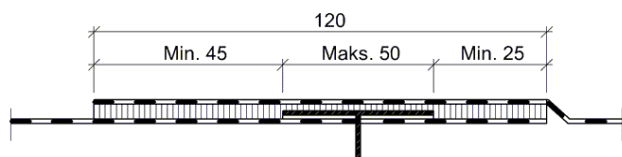
Fig. 2 Innfeste i omleggsskjøt av etlags asfalt takbelegg.
