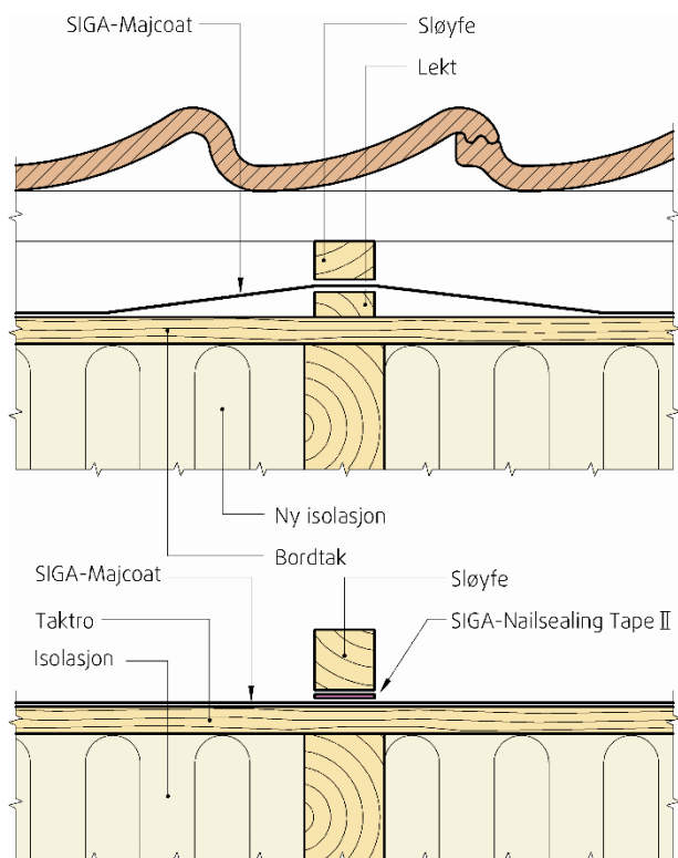
Fig. 6 SIGA Majcoat 200 lagt på taktro av bord som er isolert på undersiden. Ved ombygging av gamle tak må damptett takbelegg først fjernes. Lekt under undertaket kan brukes for å oppnå bedre sikkerhet mot lekkasjer gjennom skruehull. Lekten kan sløyfes og erstattes med SIGA Nailsealing Tape der bordtaket er plant slik at skumtapen fyller ut og tetter mellom sløyfe og bordtak.
