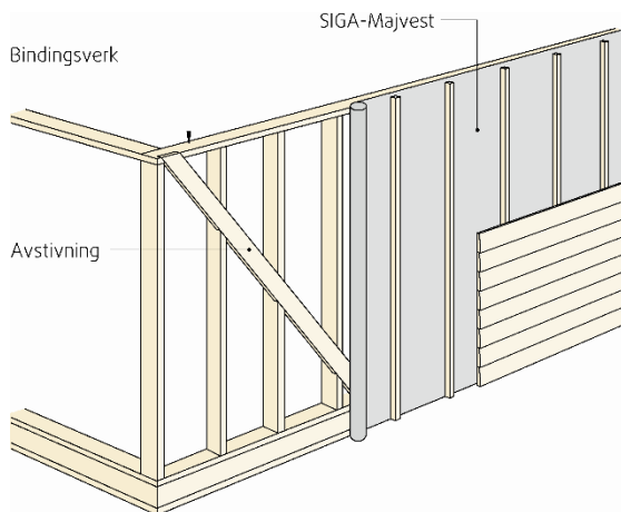
Fig. 2. SIGA Majvest 200 og SIGA Majvest 700 brukt som vindsperre på vegg. Majvest 200 med bredde 3,0 m kan legges ut i veggens høyde som vist i figuren, mens Majvest 200 med bredde 1,5 m og Majvest 700 må monteres vertikalt langs stenderne med klemte, vertikale skjøter. Det kreves egen vindavstivning av vegg.
