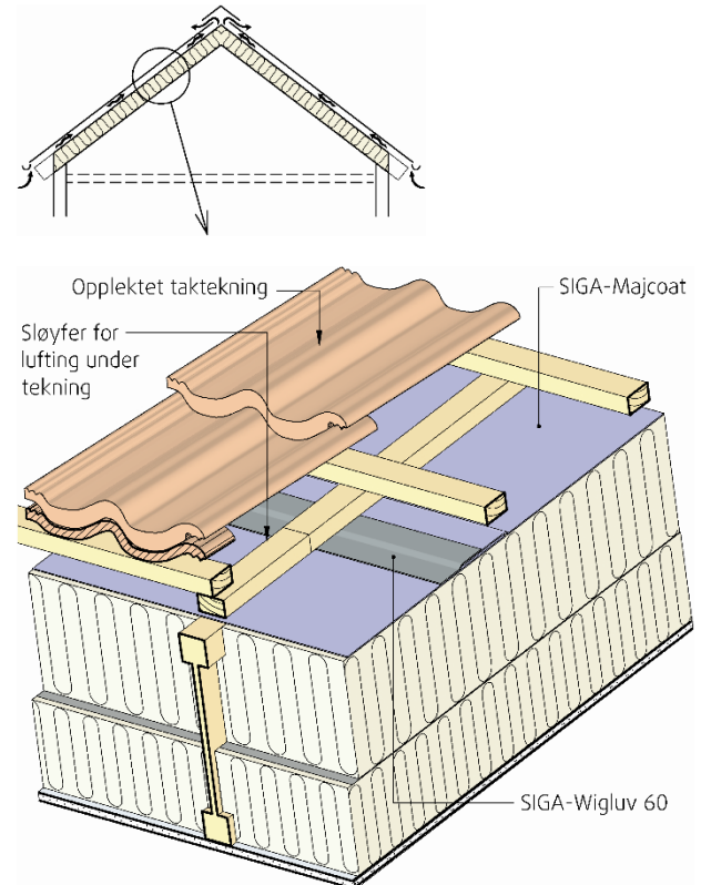
Fig. 3. Prinsipiell oppbygning av tak med SIGA Majcoat 200 kombinert undertak og vindsperre.
