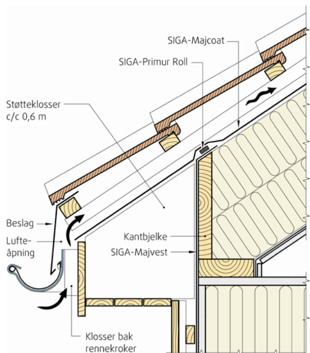
Fig. 4 Eksempel på overgang tak/yttervegg med takutstikk uten gjennomgående sperrer. Overgang mellom SIGA Majcoat og SIGA Majvest forsegles med SIGA Primur Roll.
