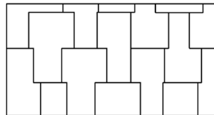
Fig. 2 Mønster til Trebolit Shingel type Rustic
