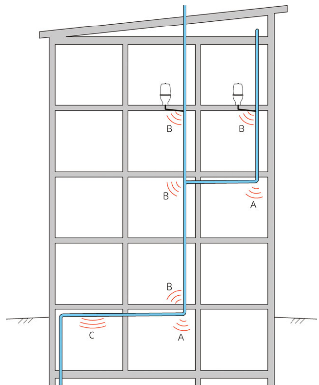
Fig. 4 Typiske monteringsituasjoner for avløpsrør. Orienterende verdier for referansesituasjonene A–C er gitt i tabell 3. Fra Byggforskeren Byggedetaljer 553.182
