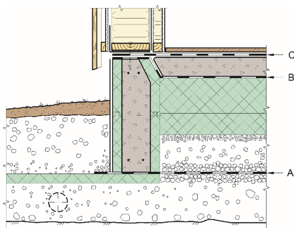
Fig. 1. Alternative plasseringer av radonmembraner
